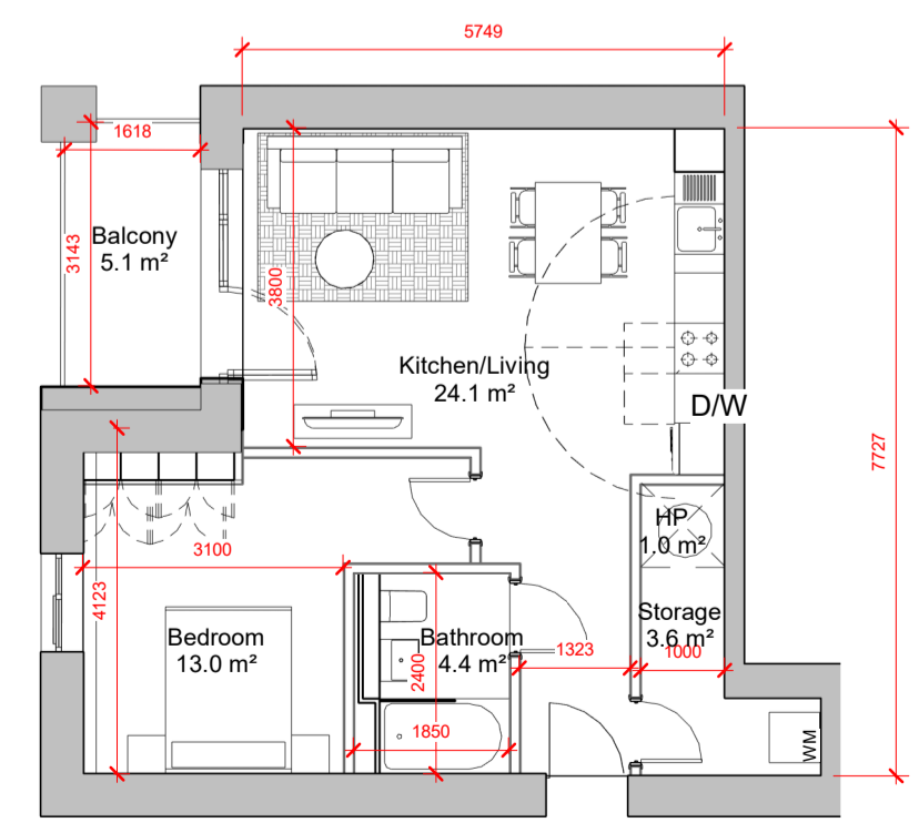
4 1 BED TYPE K 1 : 100
