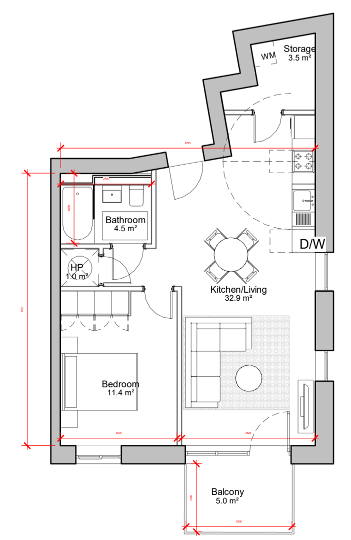
5 1 BED TYPE L 1 : 100
