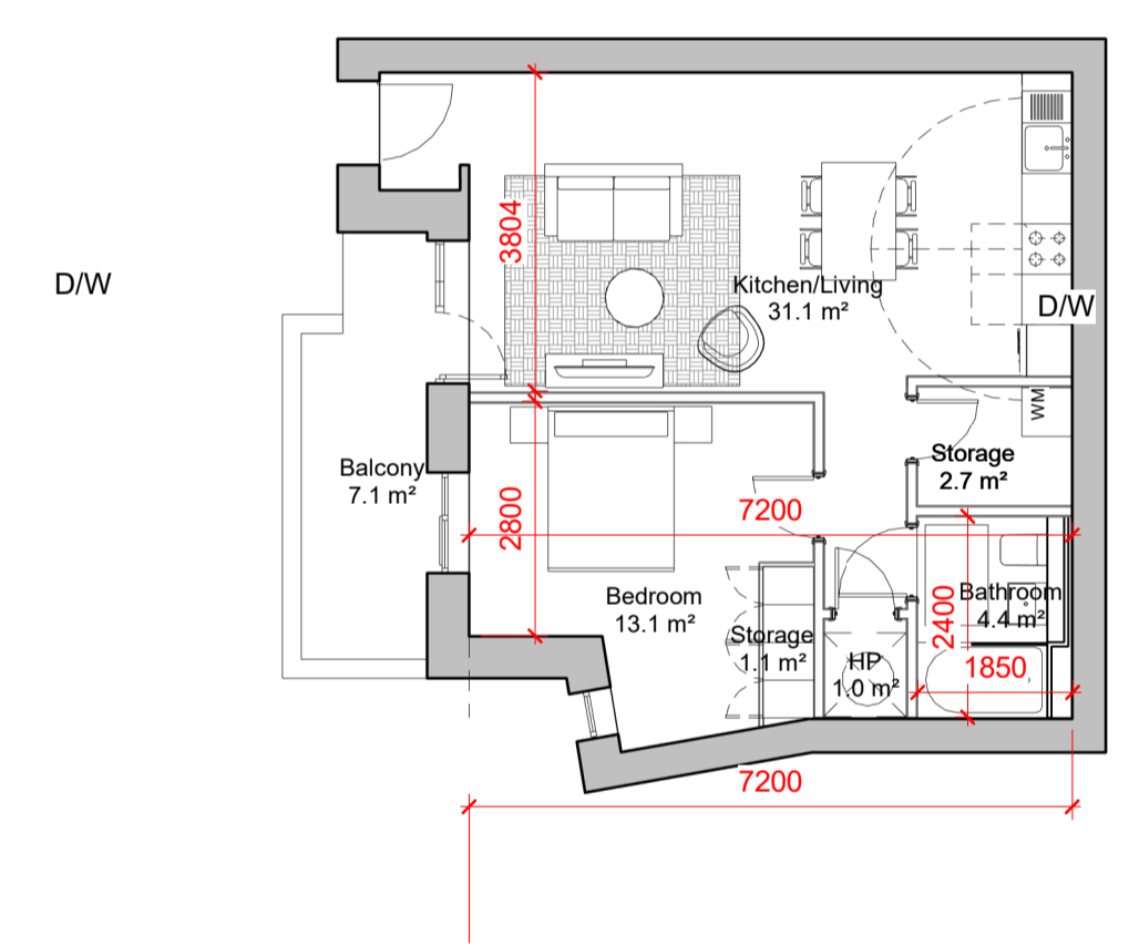
2 1 BED TYPE J3 1 : 100
