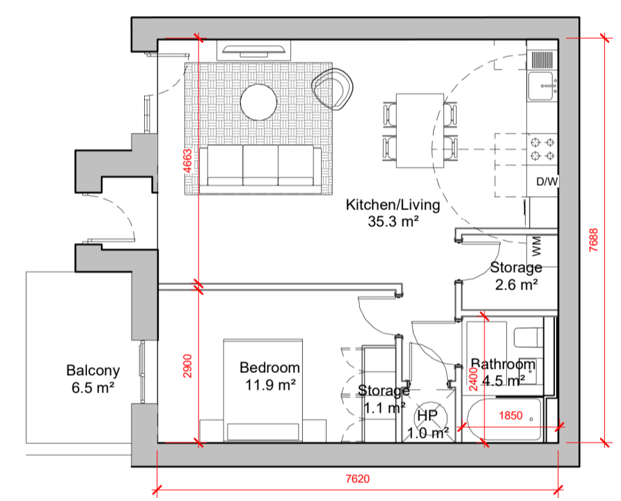
9 1 BED TYPE J 1 : 100
