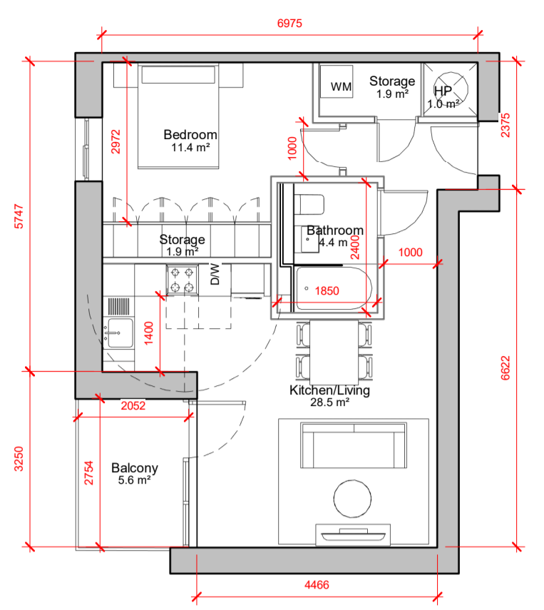
6 1 BED TYPE G 1 : 100
