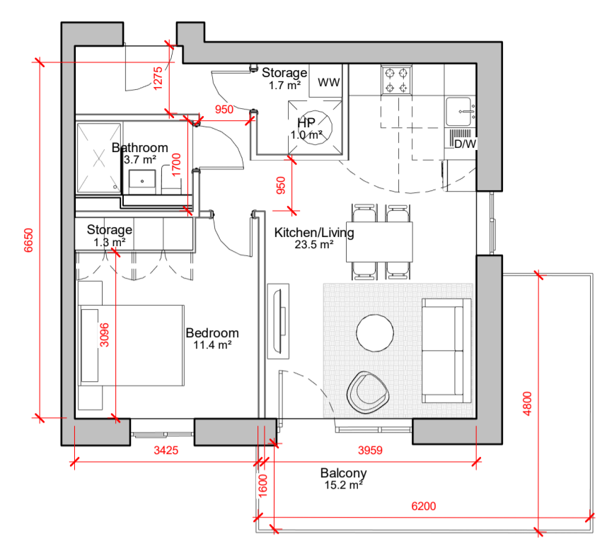
7 1 BED TYPE H 1 : 100
